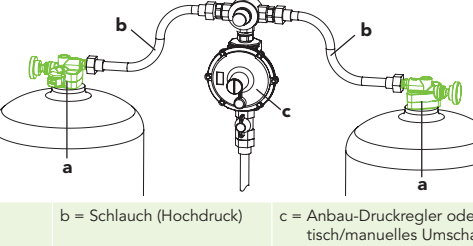
ABBILDUNG 3. STANDARD-INSTALLATIONEN - SCHNELLANSCHLUSS
